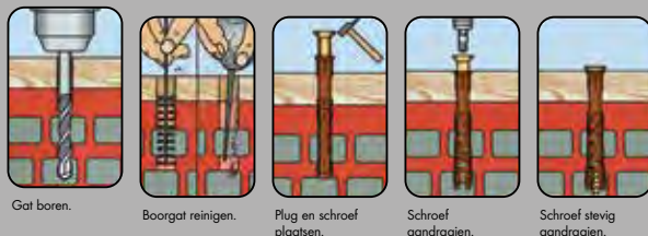
Gat boren.
