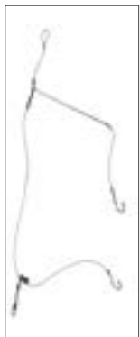
Hoofdlijn: 0,65 mm Zijlijn: 0,60 mm Lengte: 150 cm
