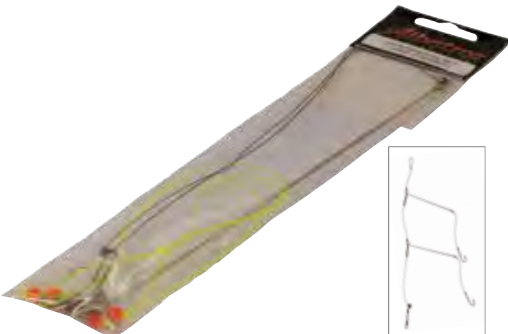
Albatros Paternoster lange afhouders Hoofdlijn: 0,70 mm Zijlijn: 0,55 mm Lengte: 105 cm
